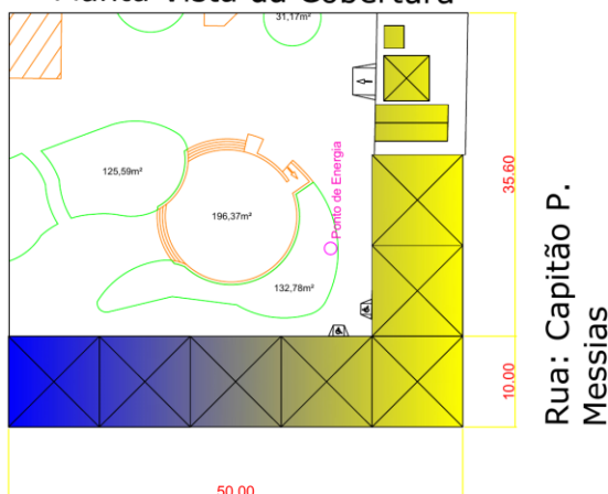
Detalhamento 01: Planta Vista da Cobertura
