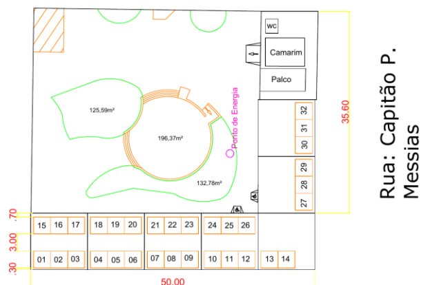
Detalhamento 02: Planta Posição das Barracas
